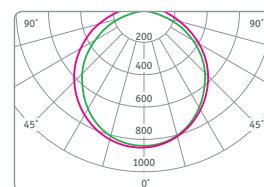
DPO-02-36-4K-IP20-LED
